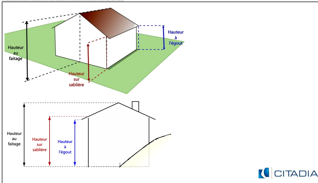
Illustration des diverses hauteurs de référence
